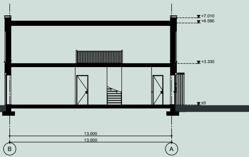
DOORSNEDE B-B
