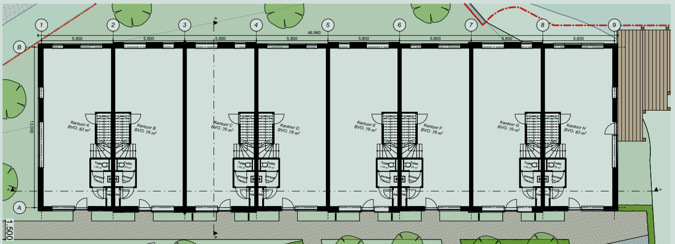
BEGANEGROND
